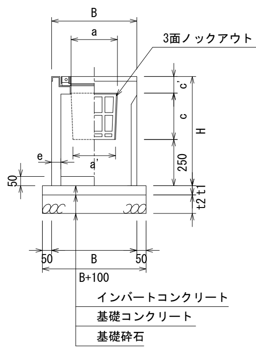
断面図
