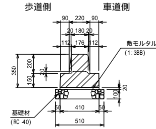
ベ - ス付歩車道境界ブロック 切下用B S=1:20
